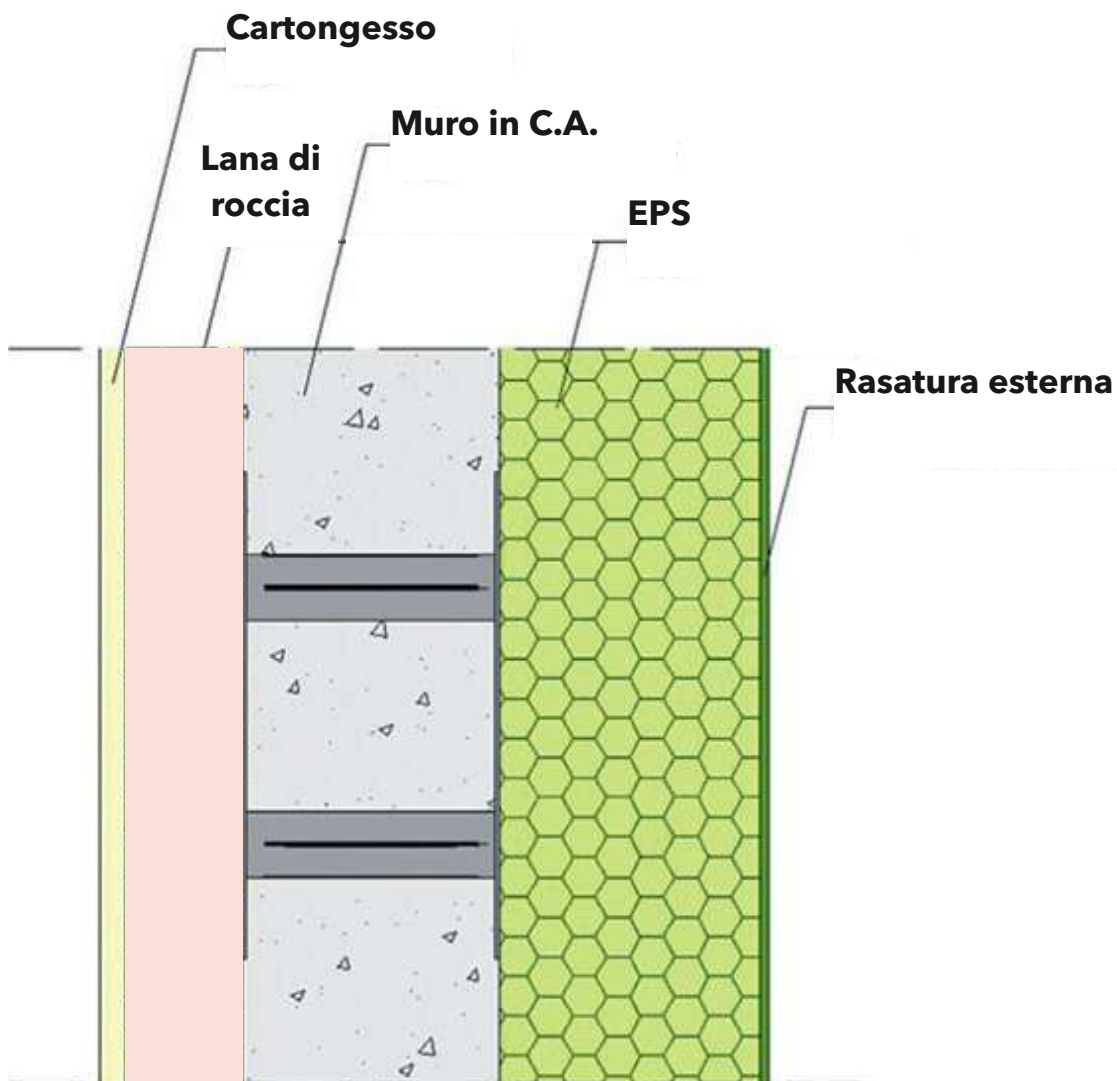
schema stratigrafico della muratura portante esterna
