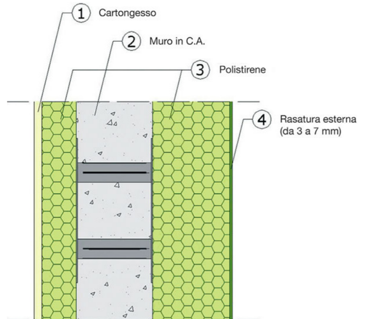
schema stratigrafico della muratura portante esterna PONTAROLO
