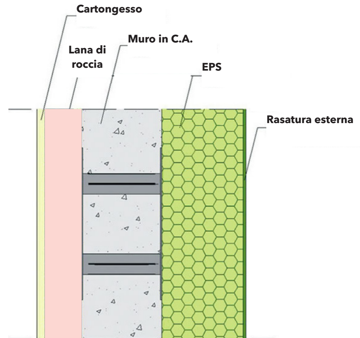
schema stratigrafico della muratura portante esterna
